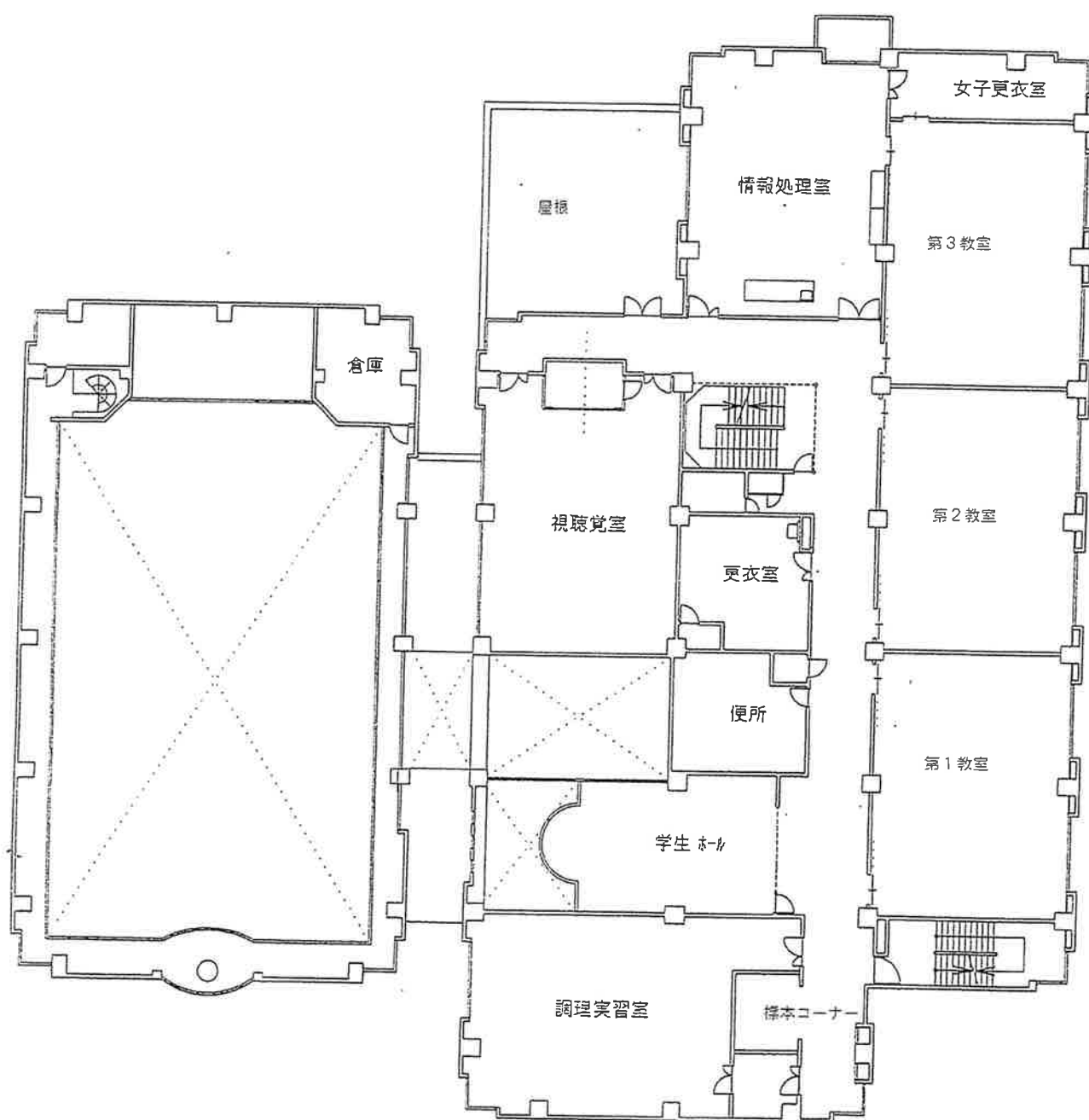
2 階 平 面 図
