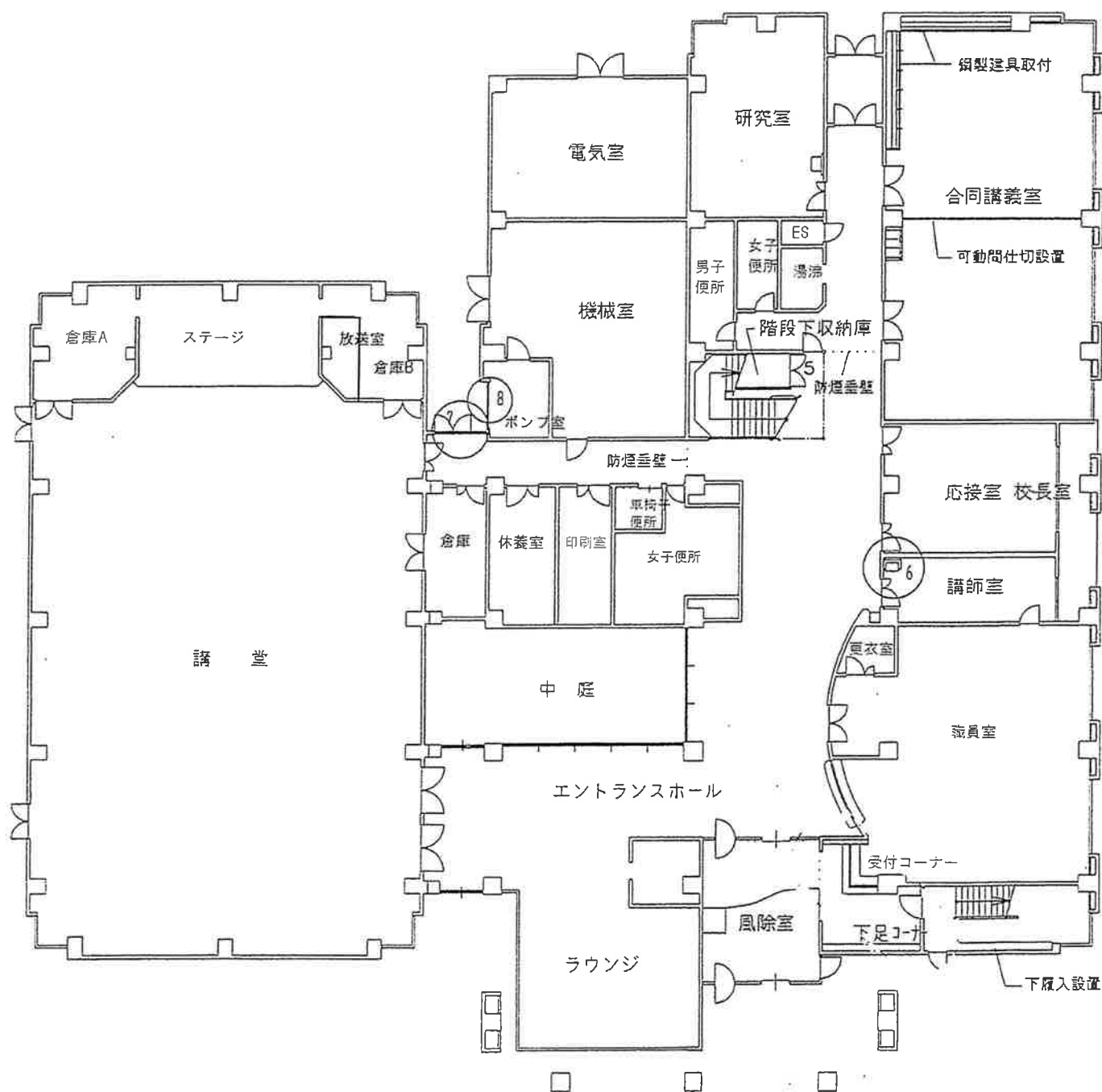
1 階 平 面 図
